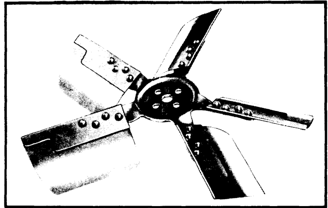
Fig. 6 Flex-Blade Fan
